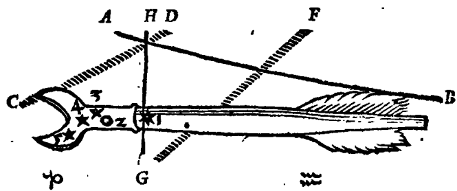
A. B. TROPICVS CANCRI C. D. F. G. EXTREMITATES LACTEAE VIAE SVNT. G. H. LINEA. PER AQVA RII INITIVM TRANSIT.
