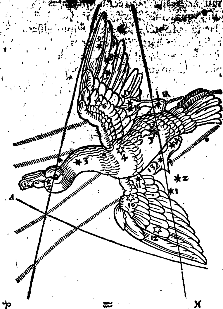
A. B. CIRCVLVS TROPICI CANCRI.
