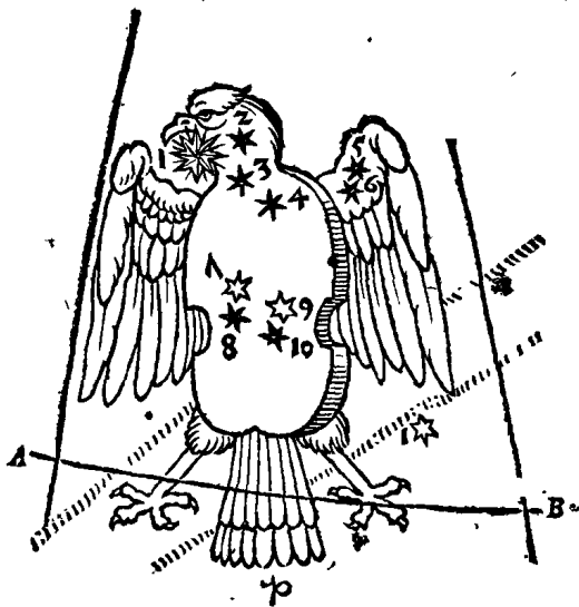
A. B. TROPICVS CANCRI.
