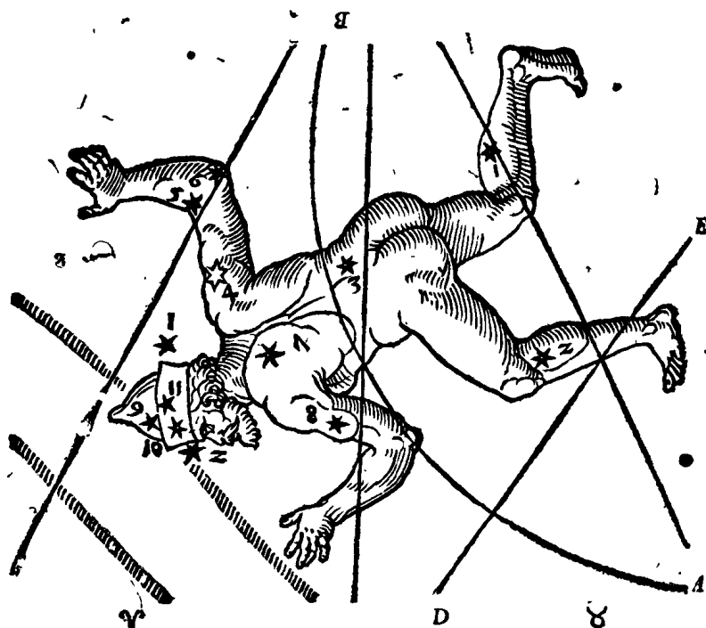
A. B. CIRCVLVS ARCTICVS. D. E. COLVRVS AEQVINOCIORVM.
