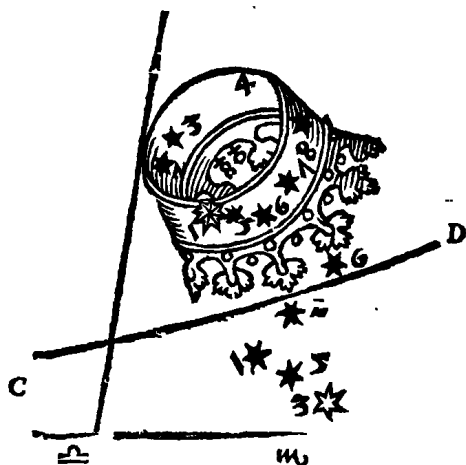
C. D. TROPICVS CANCRI.
