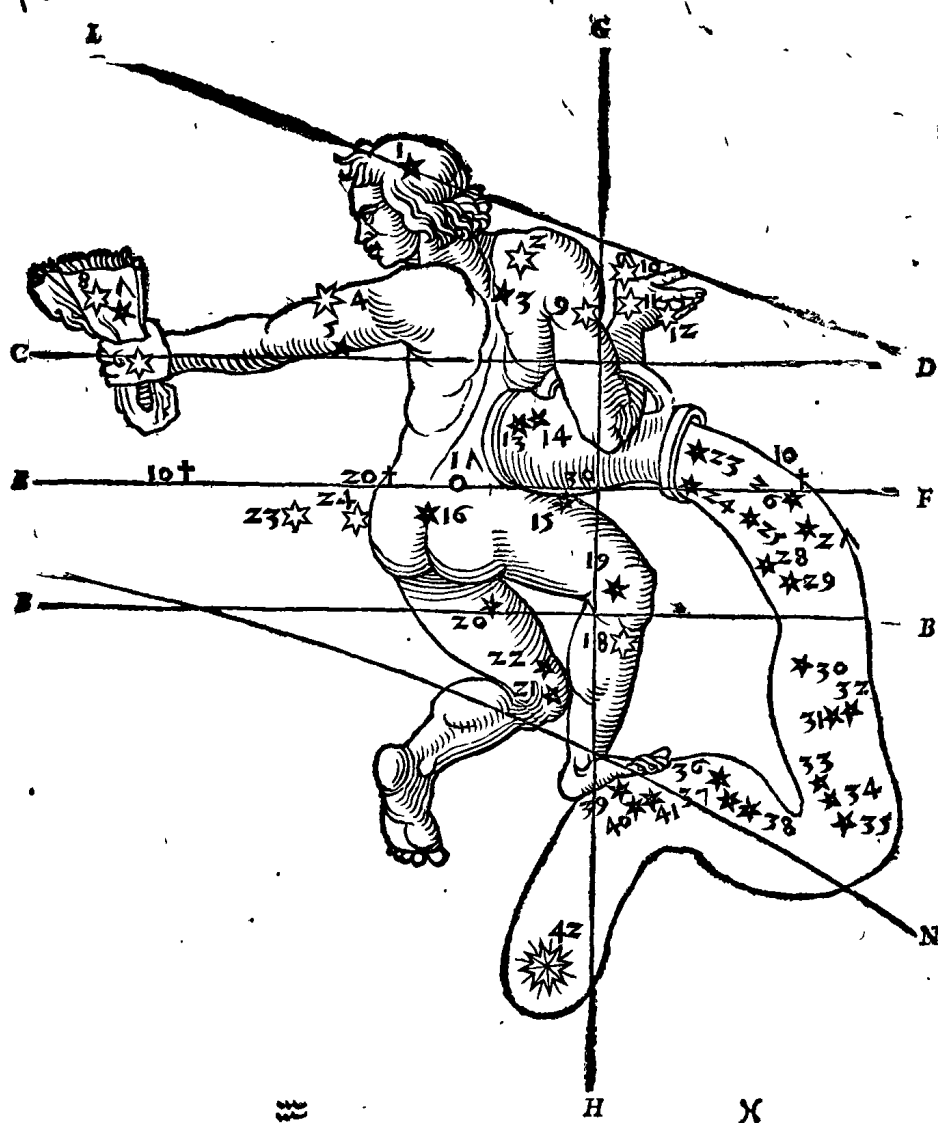
A. B. ET C. D. LIMITES AC TERMINI ZODIACI E. F. ECLIPTICA L. D. AEQVATOR. B. N. TROPICVS CAPRICORNI. G. H. LINEA, INCHOAT PISCIVM SIGNVM, ET TERMINAT AQVARIII.
