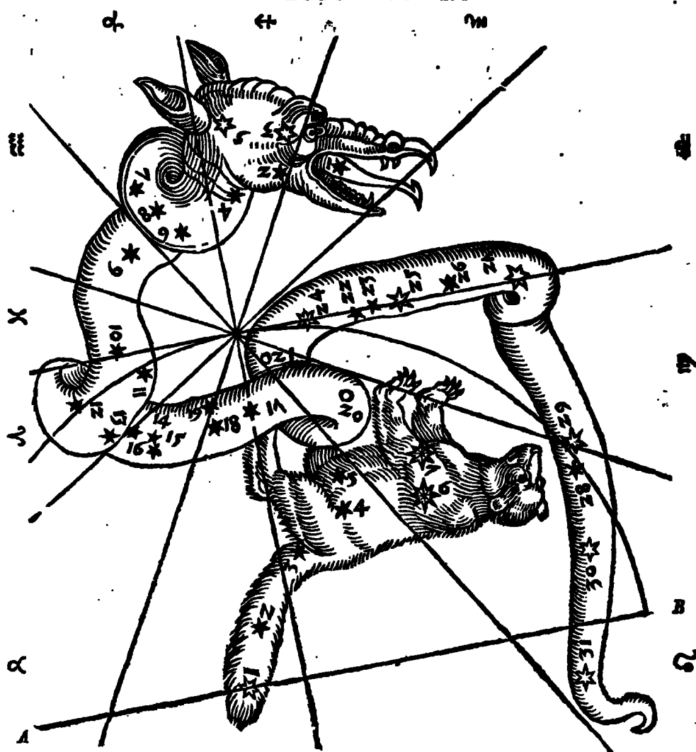
II A. B. AEQVINOCTIORVM COLVRVS.
