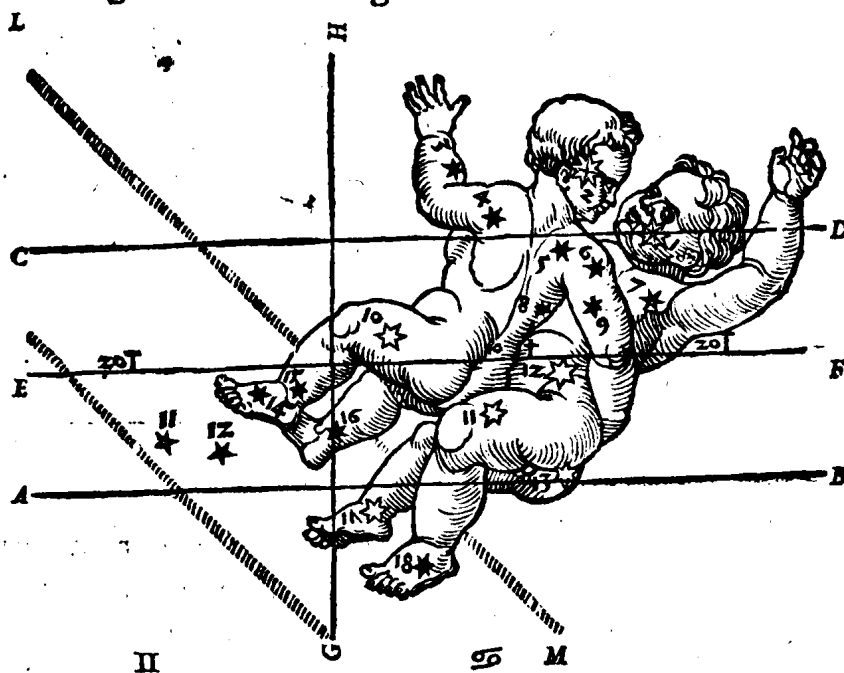
A. B. ET C. D. LIMITES ZODIACI. E. F. ECLIPTICA. L. M. ET E. G. LACTEAM VIAM NOTANT.
