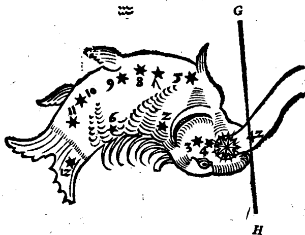
G. H. LINEA TERMINANS AQUARII SIGNVM ET INCHO- ANS DODECATEMORIVM PISCIVM
