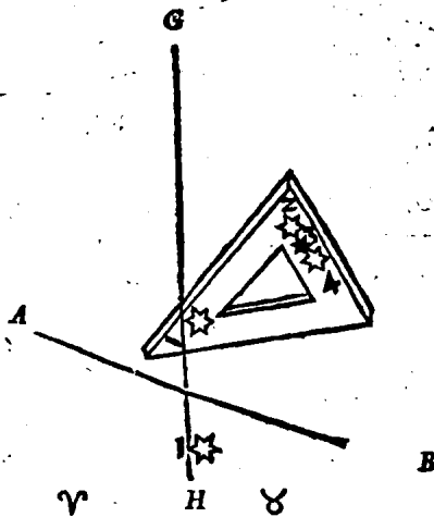
A. B. SOLSTITIALIS CIRCULI LINEA.
