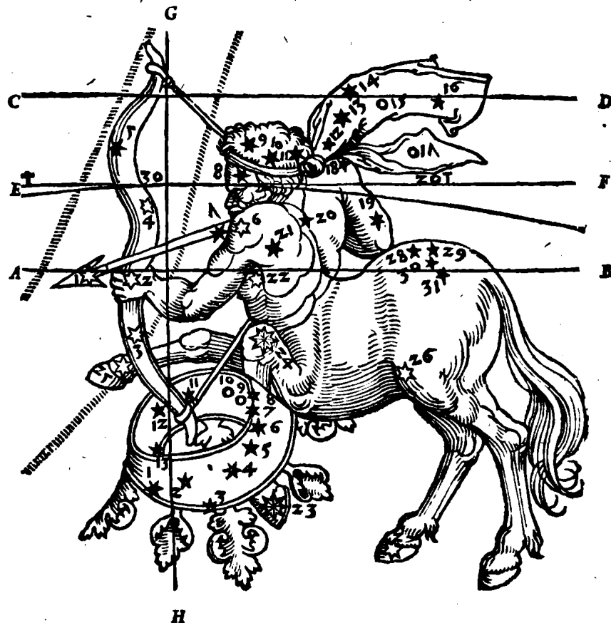
A. B. C. D. LIMITES AC TERMINI ZODIACI E. F. ECLIP- TICA. G. H. LINEA INCHOANS CAPRICORNI SIG- NVM, ET TERMINANS SAGITTARII DODECATEMORIVM.
