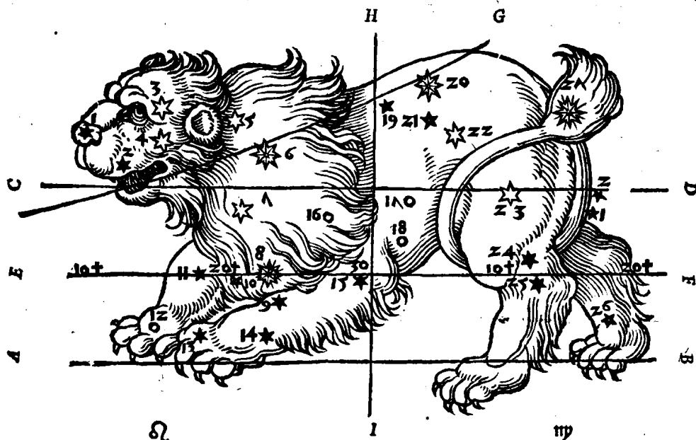
A. B. C. D. LIMITES AC ZODIACI TERMINI. E. F. SOLIS ITER. C. B. SOLSTICIALIS CIRCVLVS. H. I. DODECATEMORII LEONIS FINIS ET VIRGINIS INITIVM.
