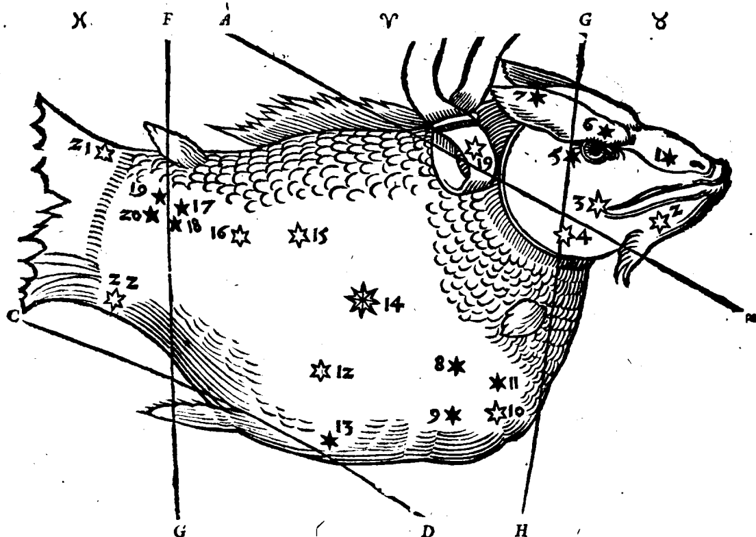
A. B. AEQVATOR. C. D. TROPICVS BRVMALIS, F. G. LINEA TRANSIENS PER FINEM PISCIVM ET ARIETIS INITIVM. G. H. TRANSIT PER FINEM ARIETIS ET TAVRI INITIVM
