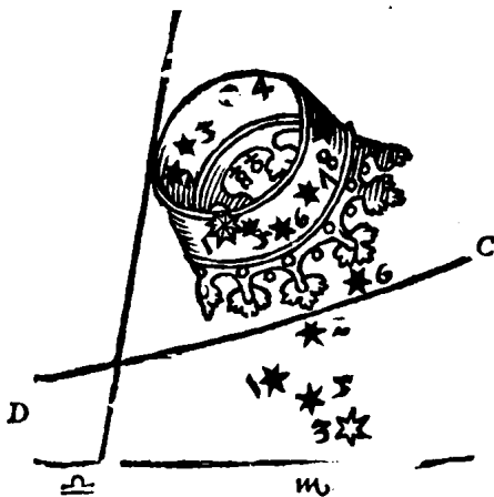
C. D. TROPICVS CANCRI.
