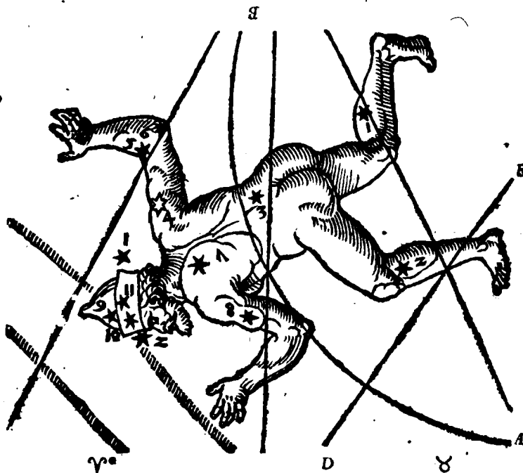
A. B. CIRCVLVS ARCTICVS. D. E. COLVRVS AEQVINOCTIORVM.
