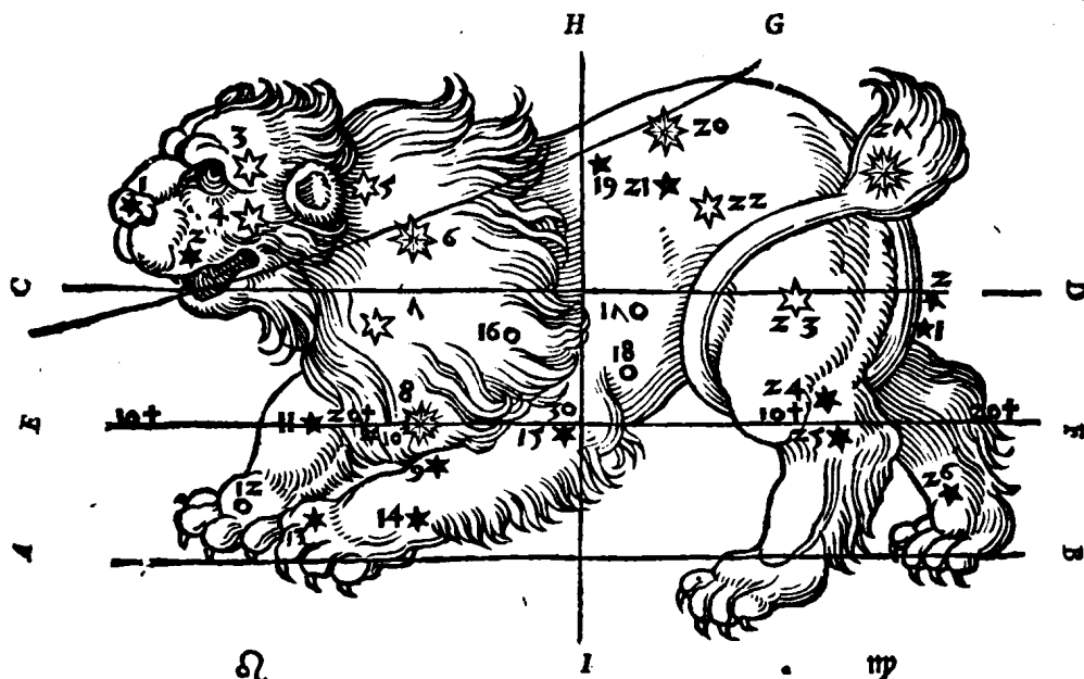
A. B. C. D. LIMITES AC ZODIACI TERMINI. E. F. SOLIS ITER. C. B. SOLSTICIALIS CIRCVLVS. H. L. DODECATEMORII LEONIS FINIS ET VIRGINIS INITIVM.
