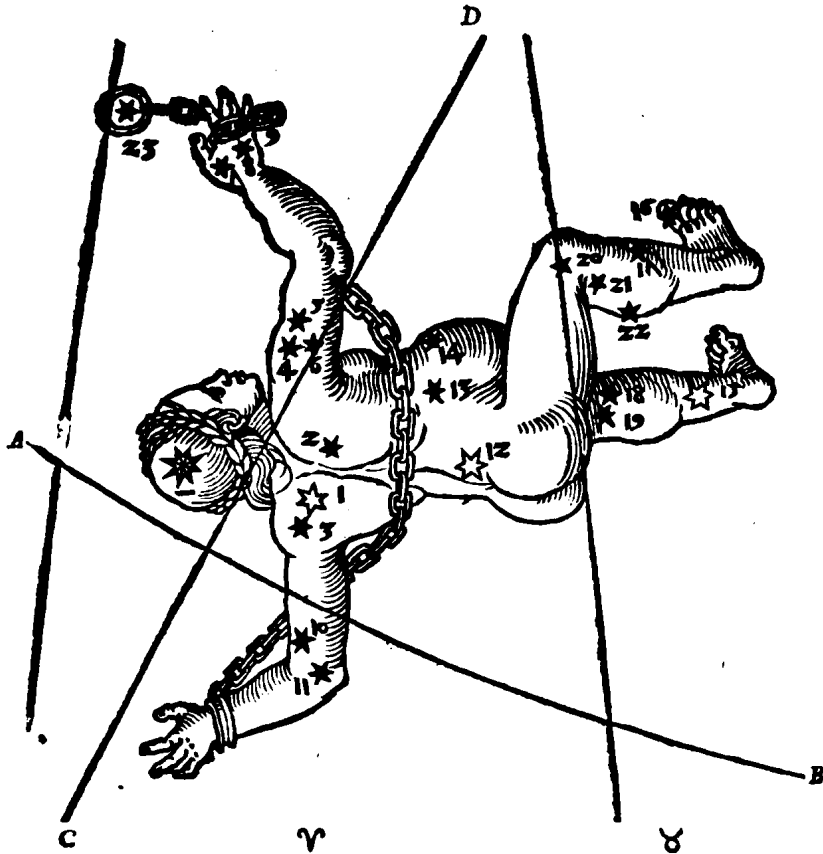
A. B. CIRCULVS AESTIVALIS LONGISSIMAM DIEM CONFICIENS. G. D. COLVRVS AEQVINOCITIA CONTINGENS.
