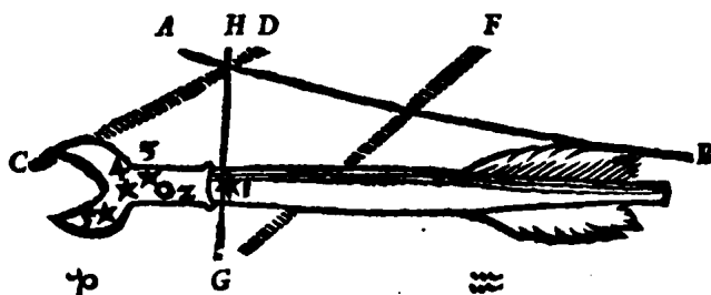
A. B. TROPICVS CANCRI C. D. F. G. EXTREMITATES LACTEÆ VIAE SVNT. G. H. LINEA. PER AQVA RII INITIVM TRANSIT.
