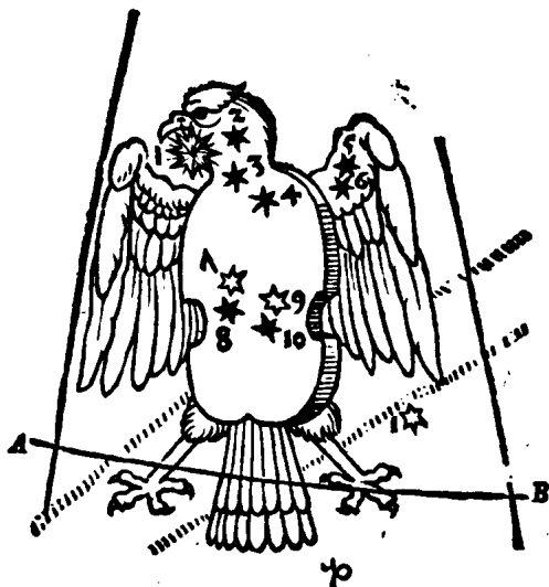
A. B. TROPICVS CANCRI.
