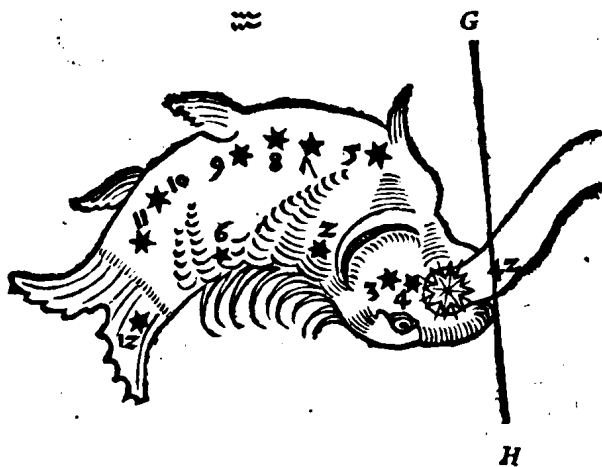
G. H. LINEA TERMINANS AQVARIJ SIGNVM ET INCHO- ANS DODECATEMORIVM PISCIVM
