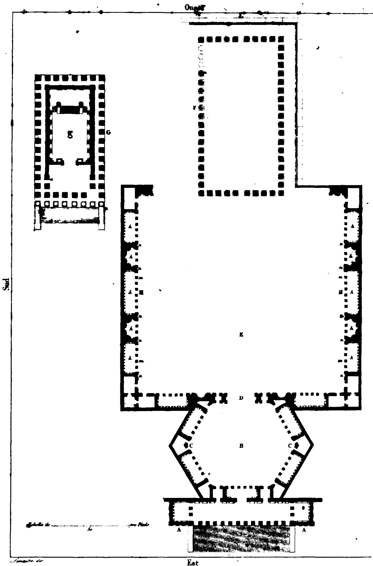
PLAN DU TEMPLE DU SOLEIL A BALBEK.
