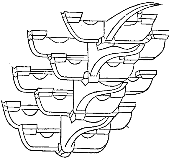
Corbeau à éperons placé sous la saillie du toit, 包. (1)
