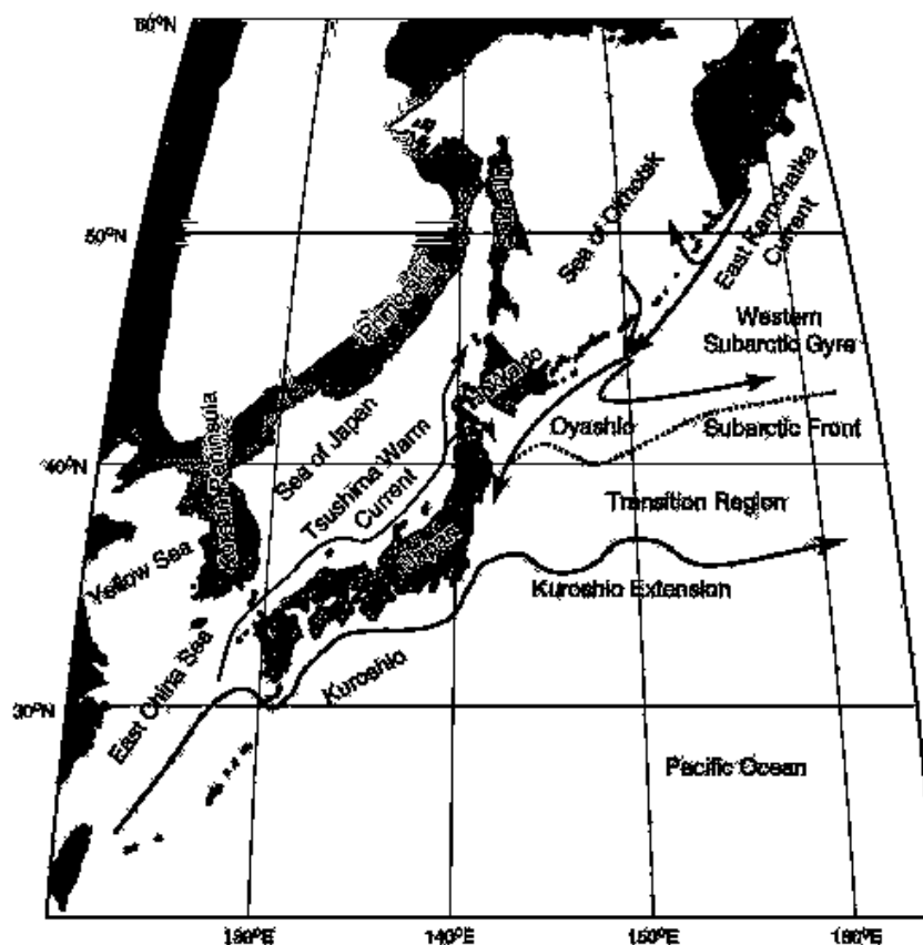
Figure 43 - Les courants dans le Pacifique
